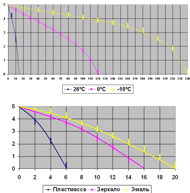
Рис. 3.7. Графики зависимости времени испарения жидкости с поверхности от времени, температуры окружающего воздуха и вида поверхности
