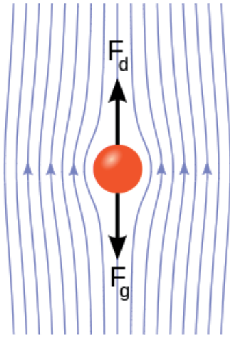
Рис. 2.7. Силы, действующие на тело, движущееся в среде
