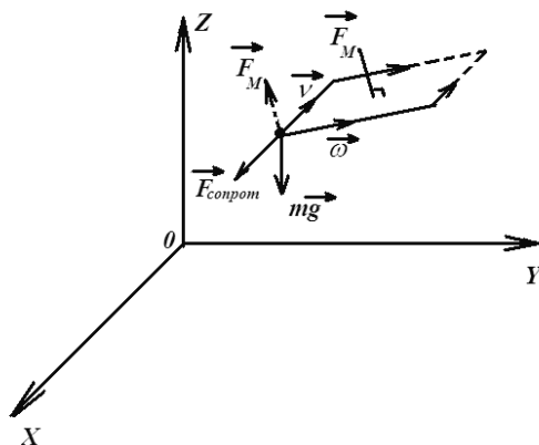
Рис. 2.6. Силы, действующие на материальную точку
